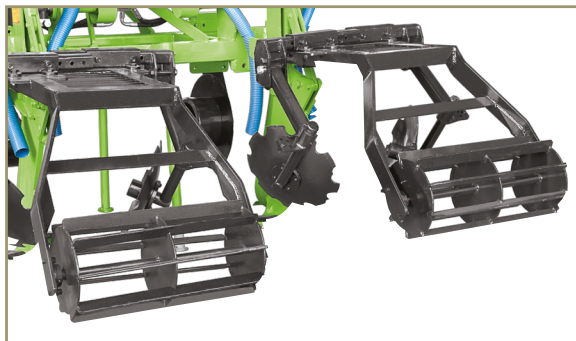
Conjunto de discos recortados e rolos niveladores.
