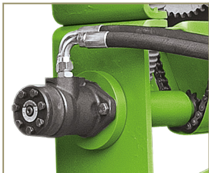
Acionamento do dosador de adubos através de motor hidráulico.
